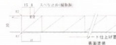
● 踏板断面図 (単位mm)
