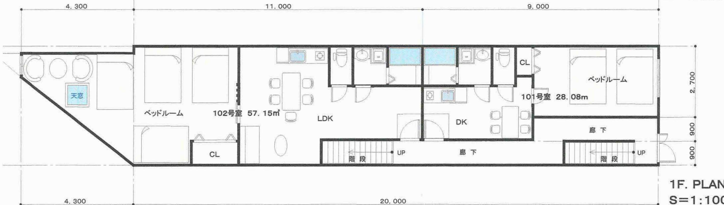
(仮称)民泊 萩ノ茶屋3丁目 PLAN S=1:100
